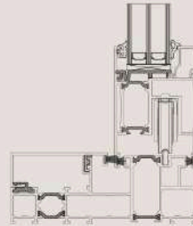
Monorail Glasdicke außen
