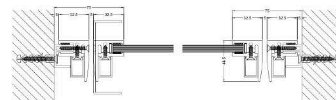
PIVOT-TÜR
