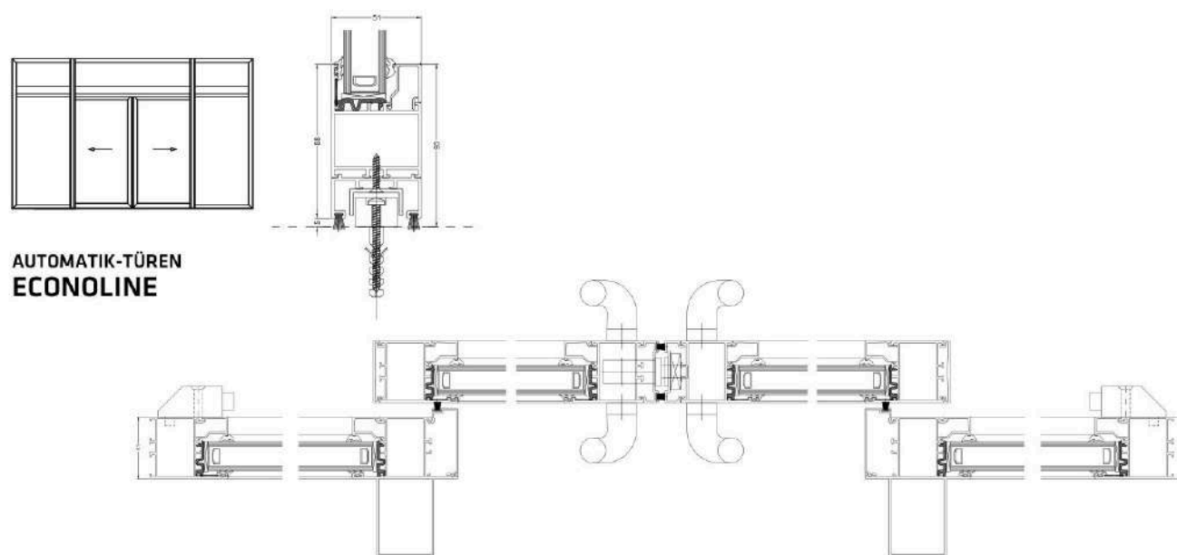
TÜR ECONOLINE
