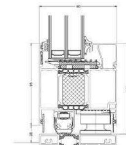
PIVOT-TÜREN STAR 90
