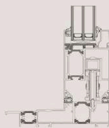
Flache Schwelle Hebe-Schiebe-System
