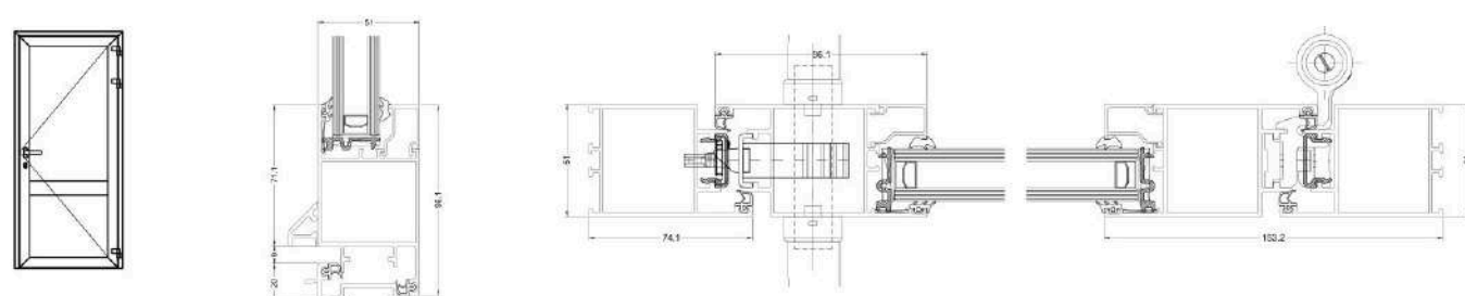
TÜR ECONOLINE
